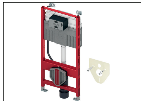
PROFIL TECE 2.0 MODUL (1016082) SUHA UGRADNJA H=112cm ZVUČ. ZAŠTITA I MONTAŽNI SET
