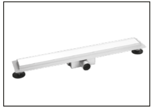
ARMAL TUŠ KANALICA 60 cm INOX (1028851) PUNA - inox, 60 x 7 cm, Fi 40/50, 35 L/min
